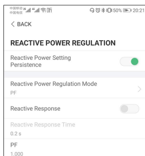
Figura 7-16 Regulação de potência reativa
