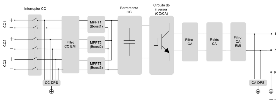
Figura 2-5 Diagrama do circuito (SG10RS-L, por exemplo)
